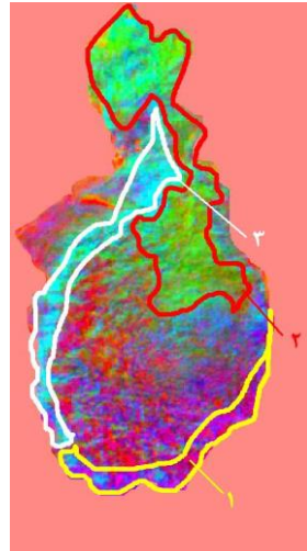
شکل ۳- ترکیب رنگی \{R: MNF2, G: MNF3, B: MNF4\} از داده های TM در محدوده VNIR+SWIR+TIR (الف) و نقشه زمین شناسی برای گنبد نمکی جهانی (بالا) و گنبد نمکی گنار سیاه (پایین) (ب)
