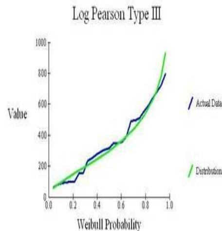
شکل ۶ دوره‌های بازگشت سیلاب‌های رودخانه زیربنه رود (منبع: نگارندگان، ۱۴۰۱)
