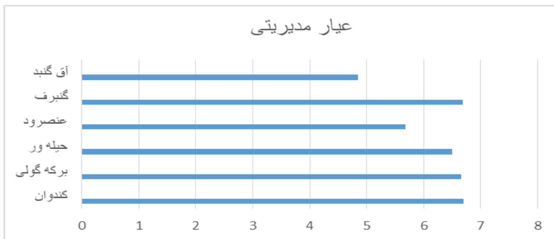
شکل ۳: نمودار امتیاز کسب شده ژئومورفوسایت ها در عیار مدیریتی در روش پیرا
