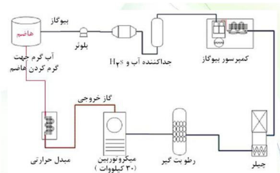
شکل شماره (۳): سیستم نیروگاه بیوگاز
